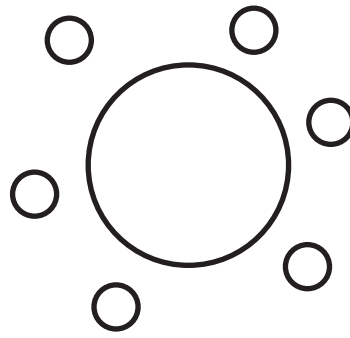
star
