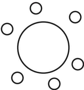
star
